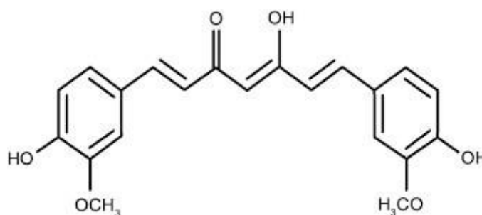
Curcumin
