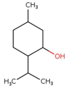
Menthol
