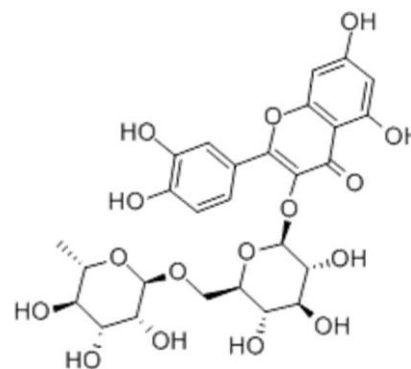
Rutin
